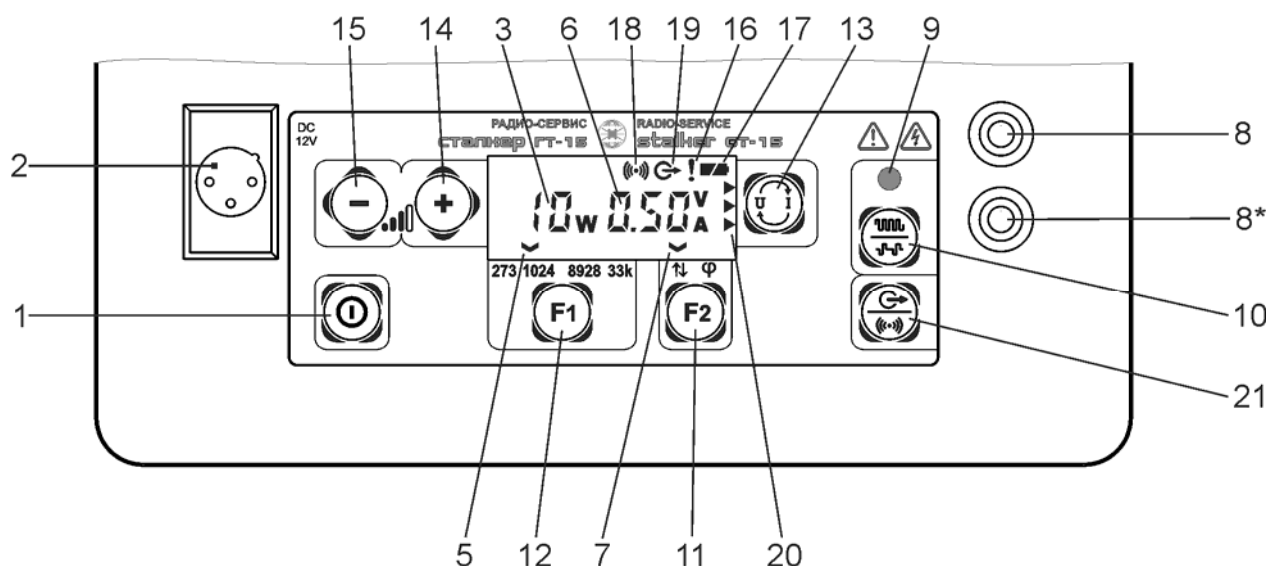
Рисунок 1.4.2 б - Передняя панель генератора ГТ-15
