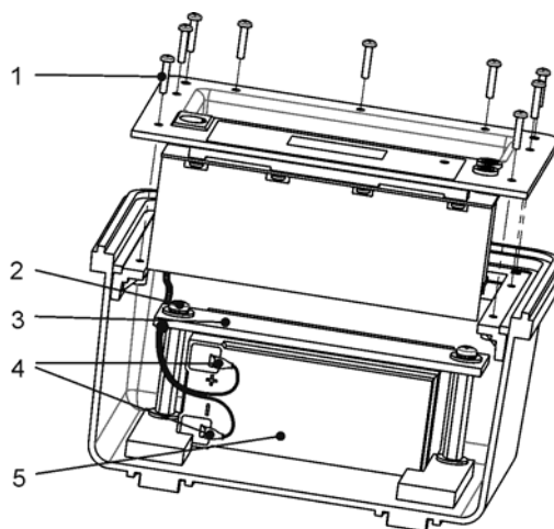
Рисунок 3.3 - Внутренняя конструкция генератора ГТ-15
