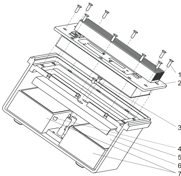
Рисунок 3.2 - Внутренняя конструкция генератора ГТ-75
