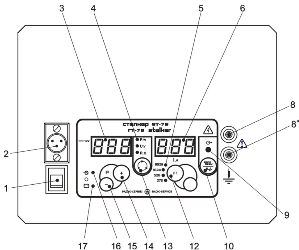
Рисунок 1.4.2 а - Передняя панель генератора ГТ-75
