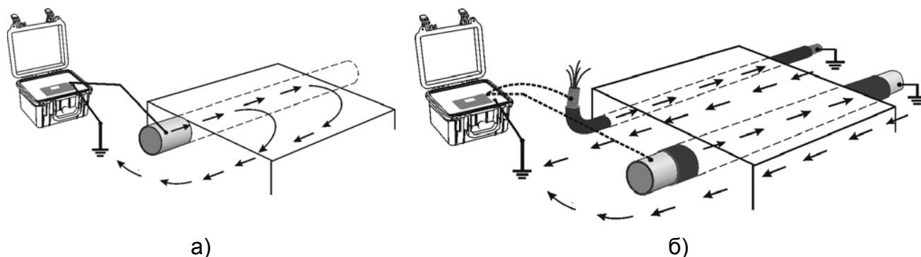
Рисунок 2.3.1 –Подключение генератора к коммуникациям:
