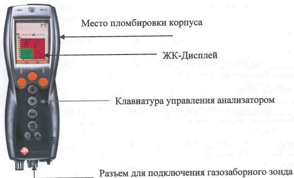
Рис. 1. Testo 330
