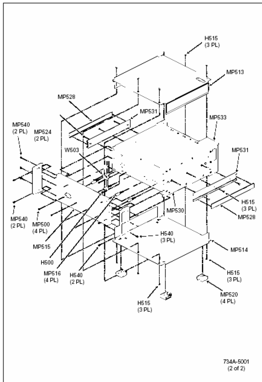
Рисунок 6-1. Эталон постоянного напряжения 734A (продолжение)
