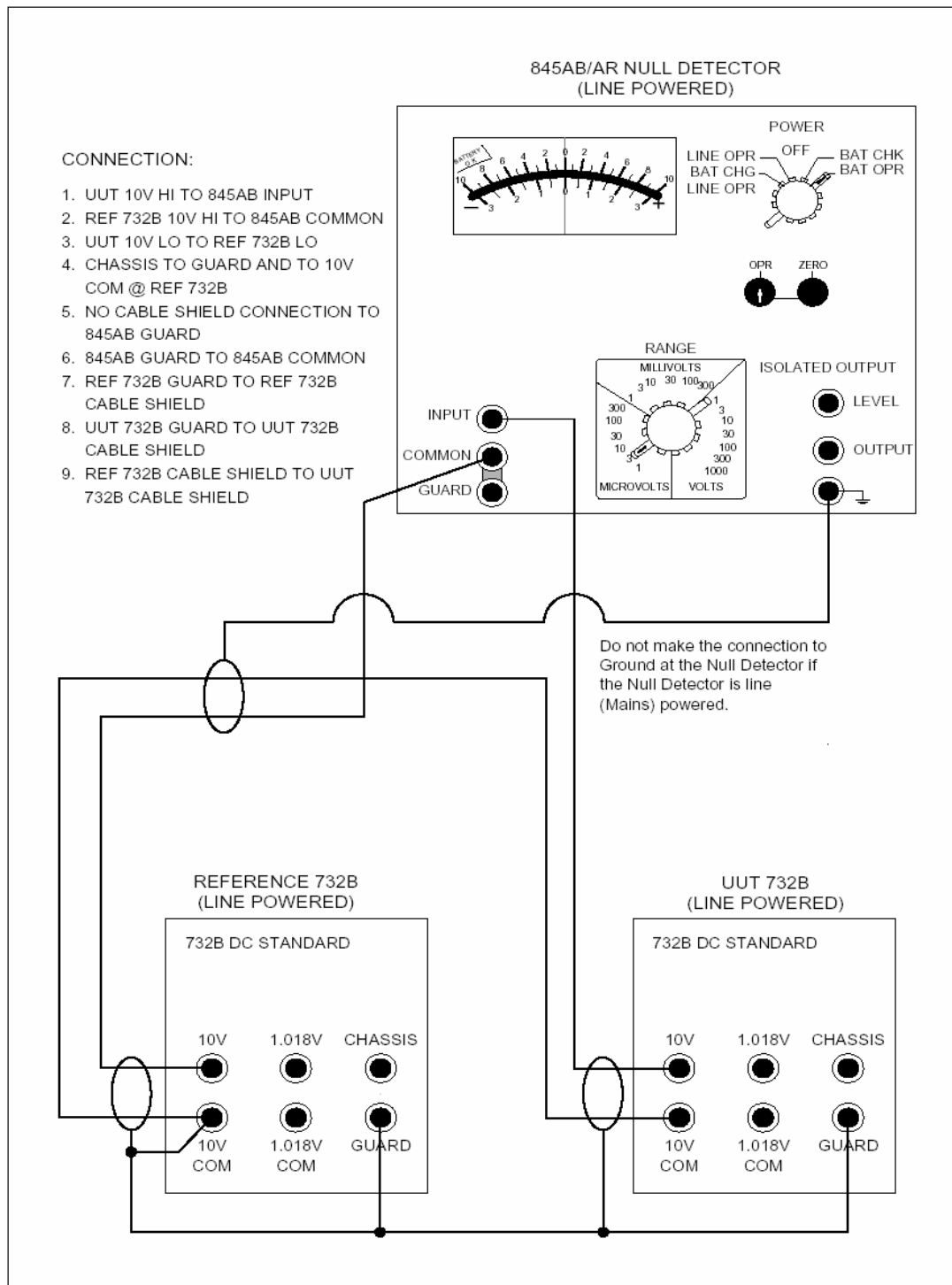
Рисунок 5-1. Соединения при калибровке выхода 10V
