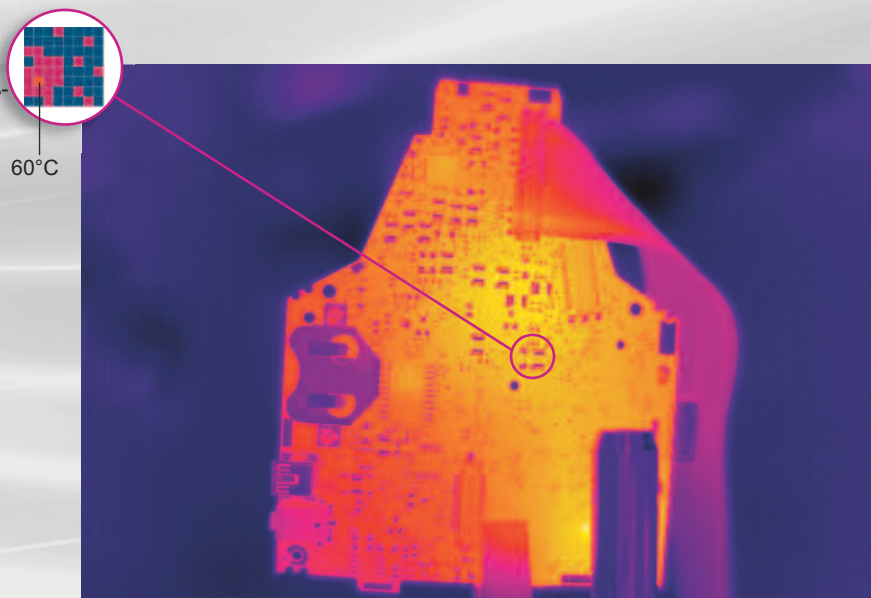
Термограмма в мегапиксельном качестве, созданная с помощью технологии SuperResolution —> 1280 x 960 пикселей
