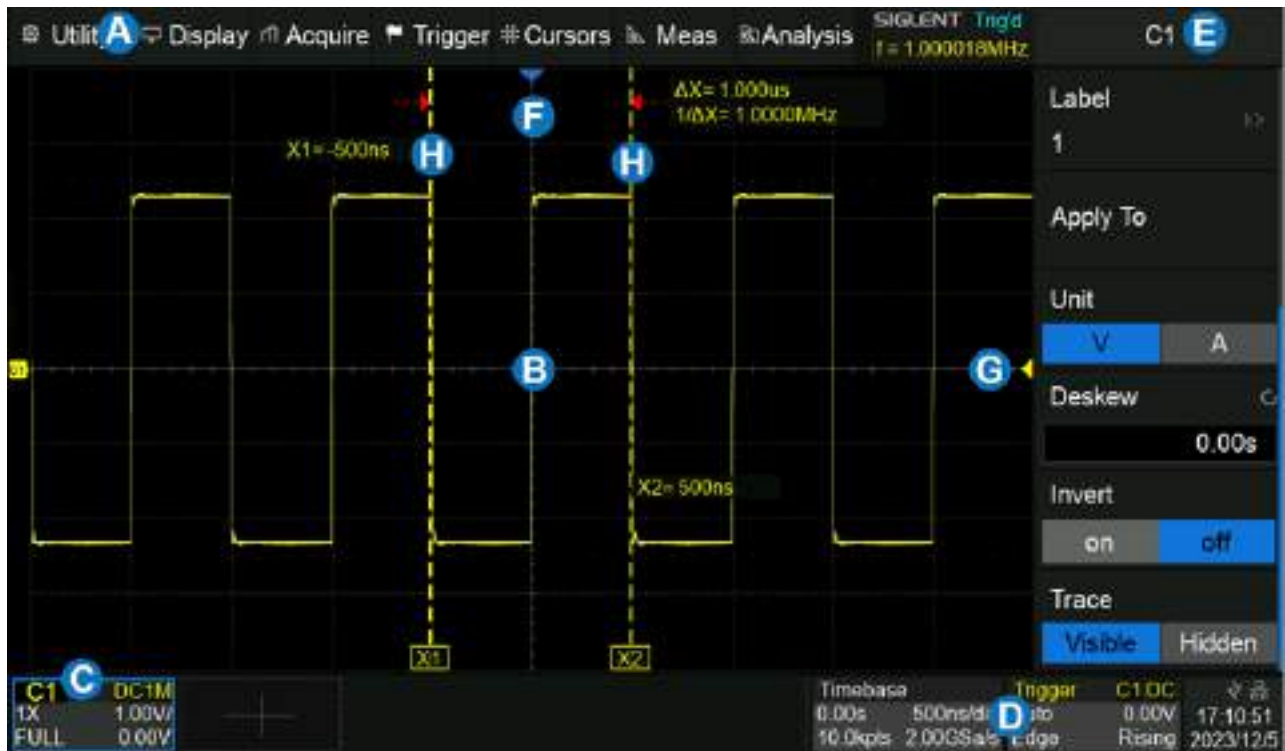
Рис. 10-1 Окно осциллографа сери АК ИП-4149
