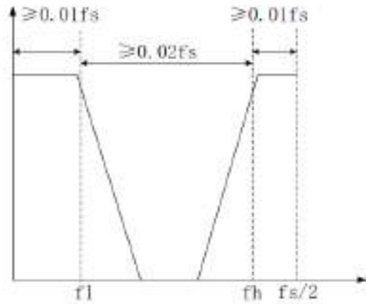
Режекторный фильтр
