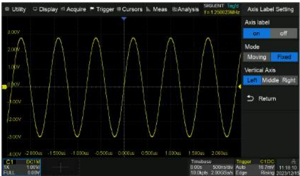
Рис. 28-2 Фиксированный режим
