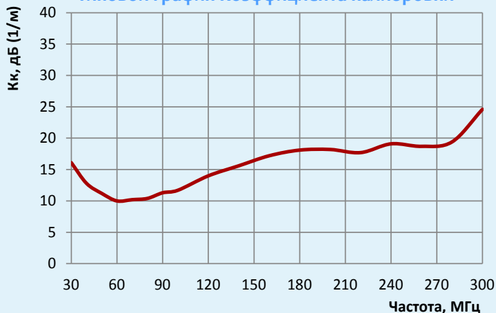
Типовой график Коэффициента калибровки
