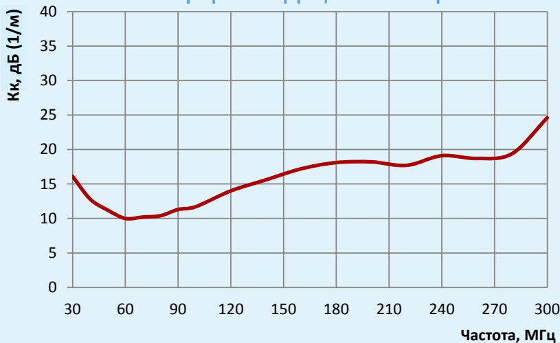
Типовой график Коэффициента калибровки
