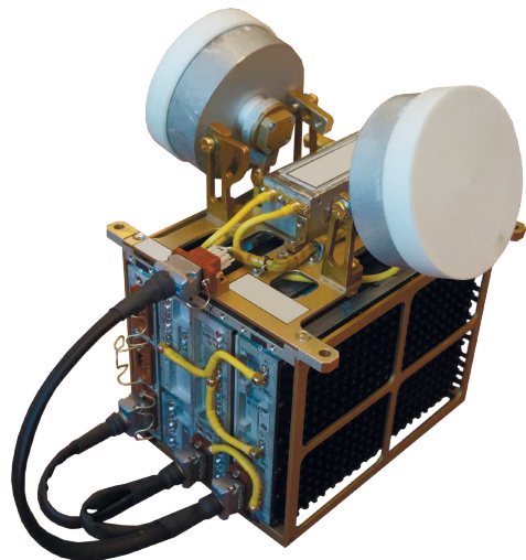
На фото: 2-канальный преобразователь частоты диапазона 0,9-18 ГГц, серии Универсал – 1, комплексированный с антенной системой
