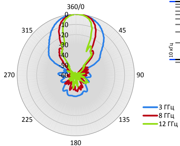
График ДН
