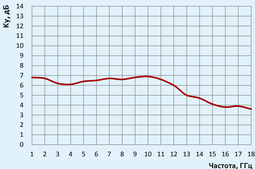
Типовой график K_u
