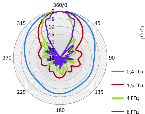
График ДН
