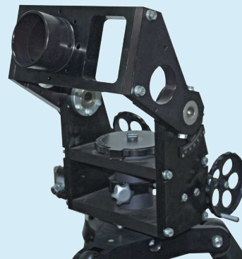
На фото: Опорно-поворотное Устройство (ручное).
