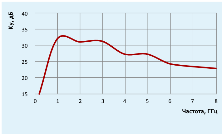
Типовой график Коэффициента усиления с МШУ
