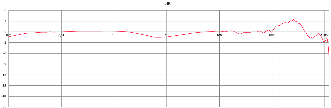
RSS2010A Типичное значение АЧХ
