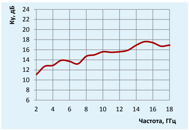
Типовой график Коэффициента усиления
