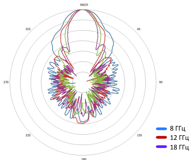
График ДН
