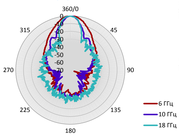
График ДН
