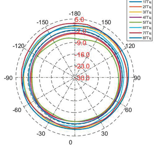
График ДН
