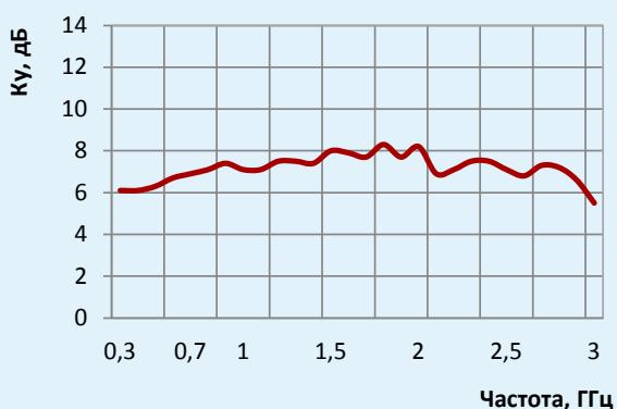
Типовой график Коэффициента усиления
