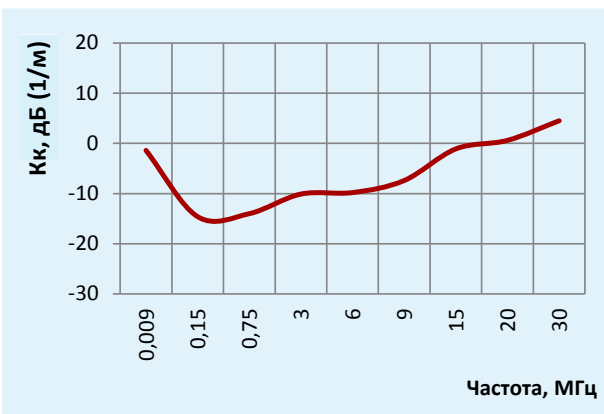
Типовой график Коэффициента калибровки
