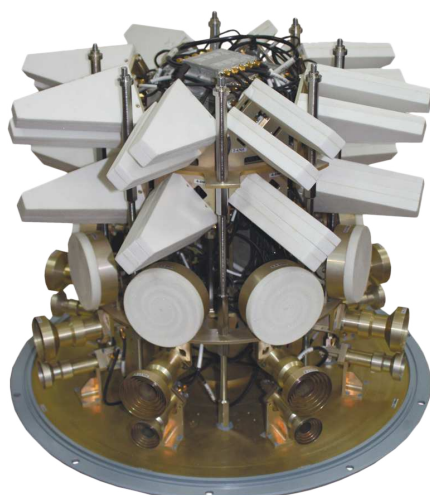
АСКМ 5/8-0,9/18
