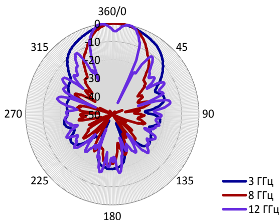
График ДН
