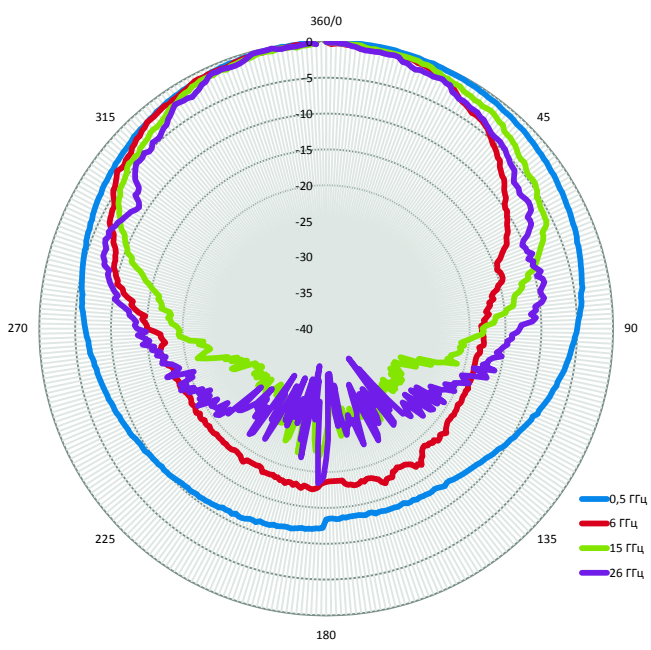
График ДН
