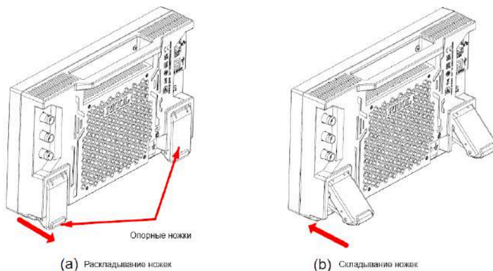
Рисунок 5.1 Выдвижение и складывание опорных ножек
