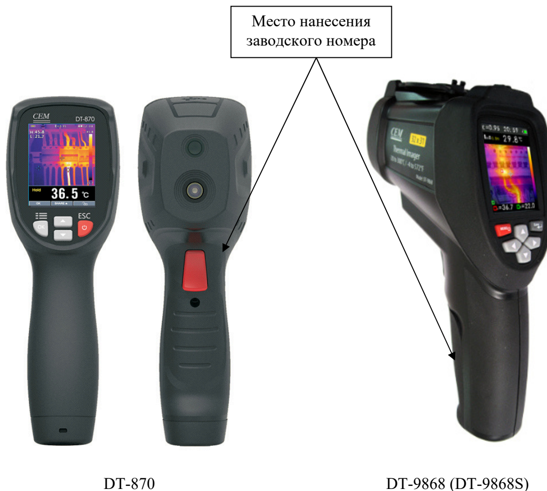
Рисунок 1 - Общий вид тепловизоров инфракрасных DT-870, DT-9868
