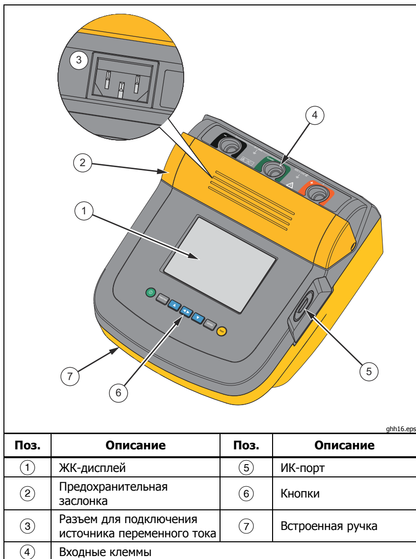
Рисунок 2. Измеритель сопротивления изоляции 1550C/1555
