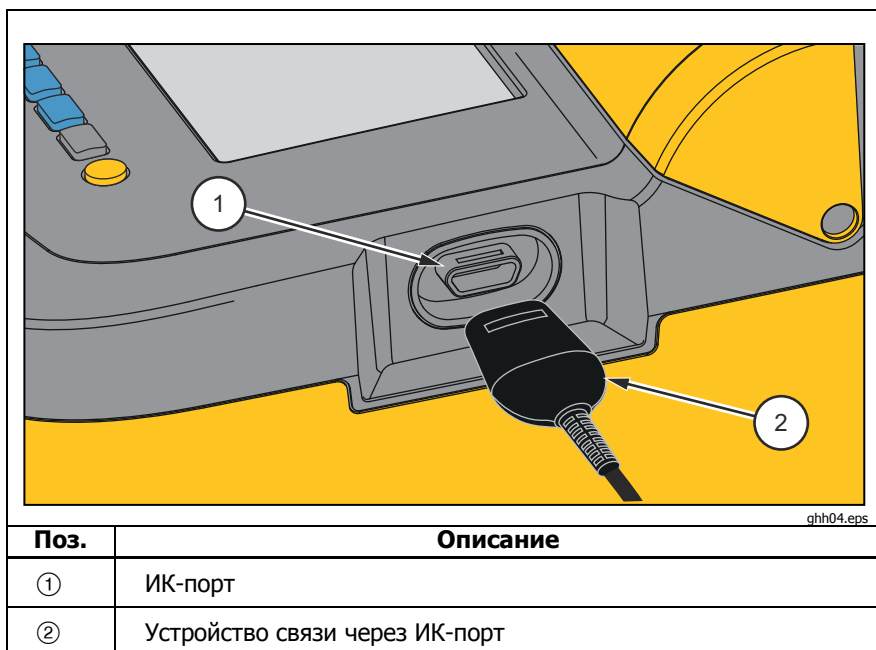
Рисунок 13. ИК-порт на измерителе сопротивления изоляции 1550C/1555
